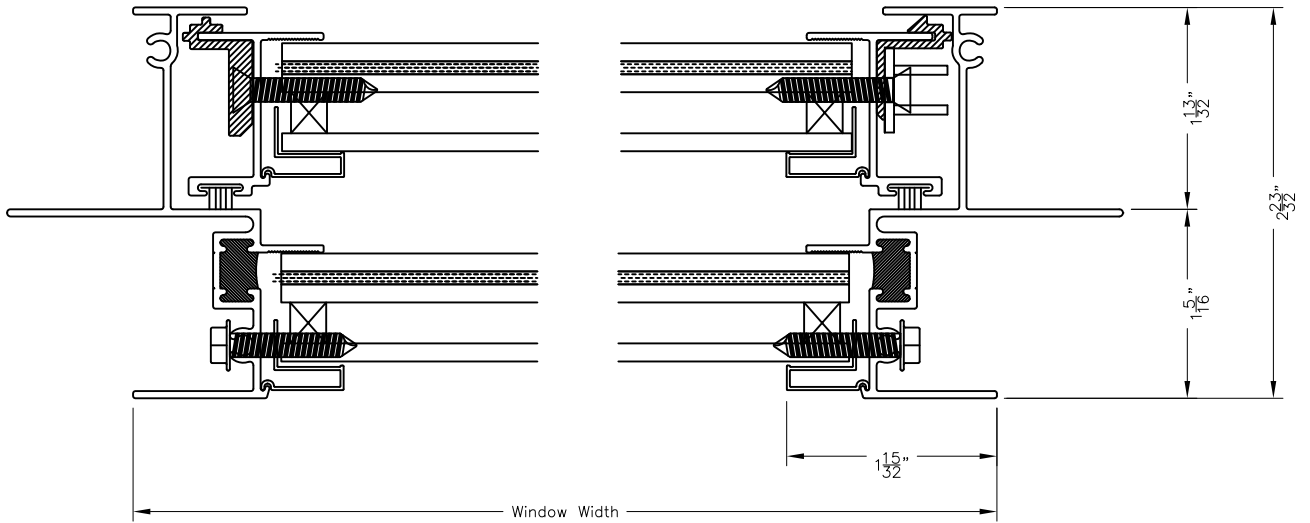
SECTION B-B SCALE: 3:4
